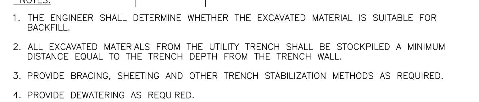
D15 2 PIPE TRENCH DETAIL – PAVEMENT N.T.S.
