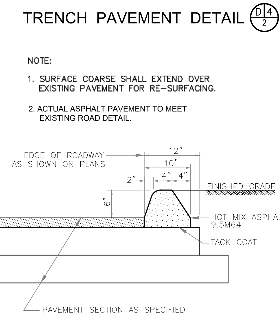
HOT MIX ASPHALT CURB DETAIL N.T.S.
